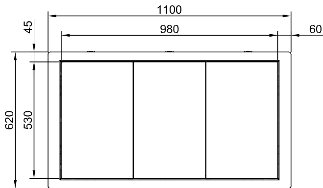
Boven aanzicht
